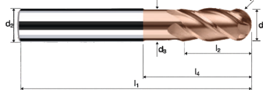
H7490 Schnittdaten: Fraisa Katalog Hochleistungs-Fräswerkzeuge 2021 - Seite 338
