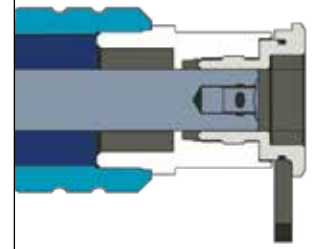
Kolbenstange eingezogen
