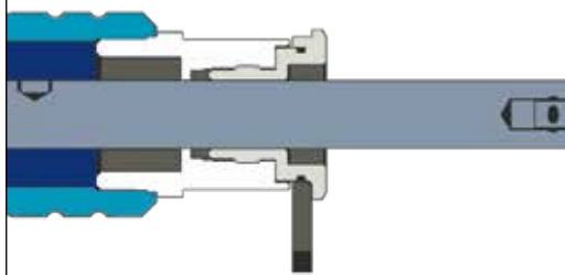
Kolbenstange ausgeschoben
