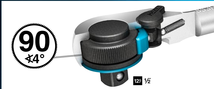
90 Zähne, 4° Schwenkwinkel
