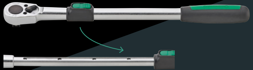
5-fach verstellbarer Teleskopauszug
